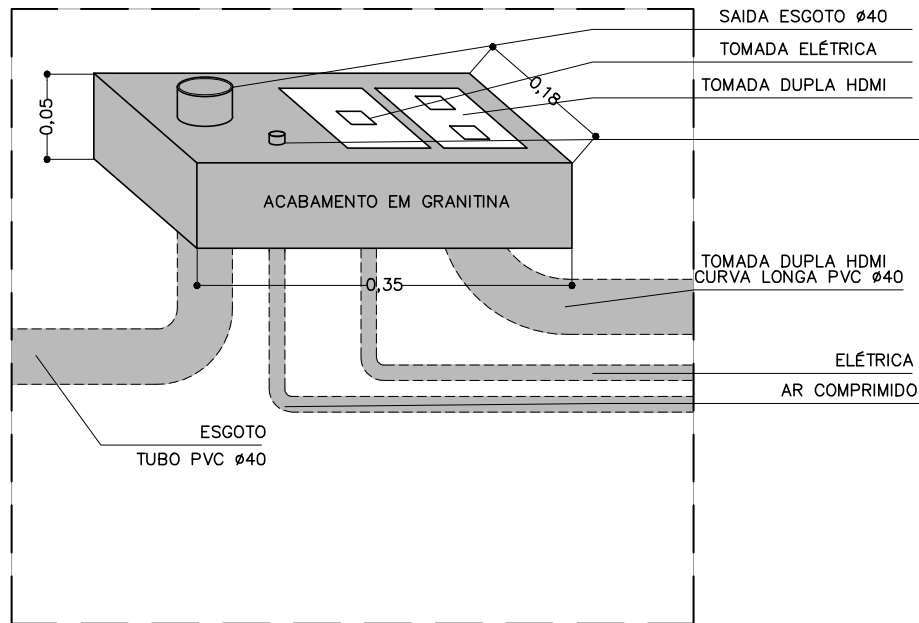
DETALHE DO SÓCULO DA BANCADA DO PROFESSOR SEM ESCALA
