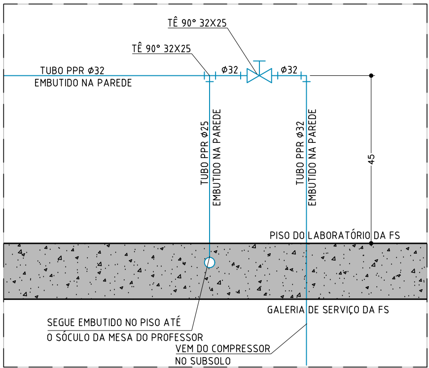
DETALHE DO REGISTRO GERAL ESCALA 1/10
