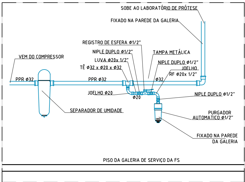
DETALHE DO PURGADOR AUTOMÁTICO SEM ESCALA
